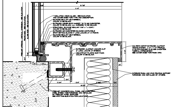
B PERIMETER FRAME DETAIL SCALE: 2" = 1'-0"
