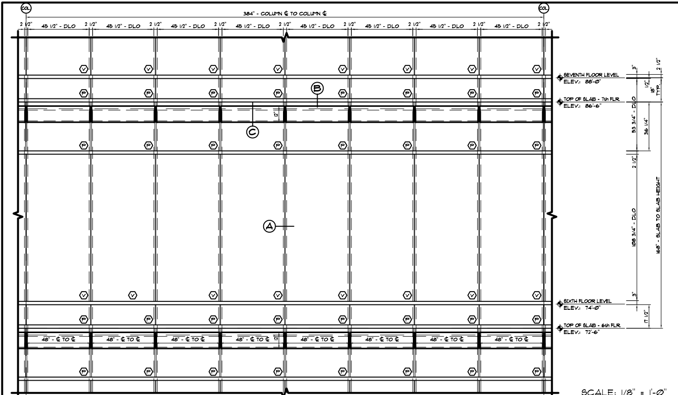
SCALE: 1/8" = 1'-0"
