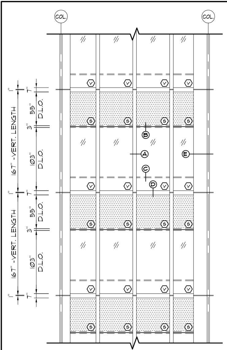
SCALE: 1/8" = 1'-0"
