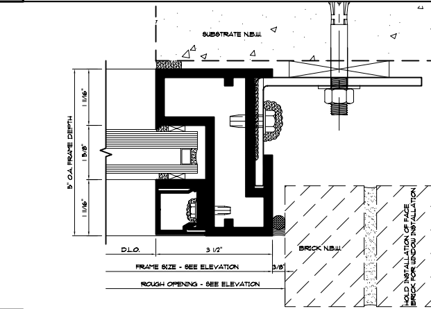
D JAMB DETAIL
